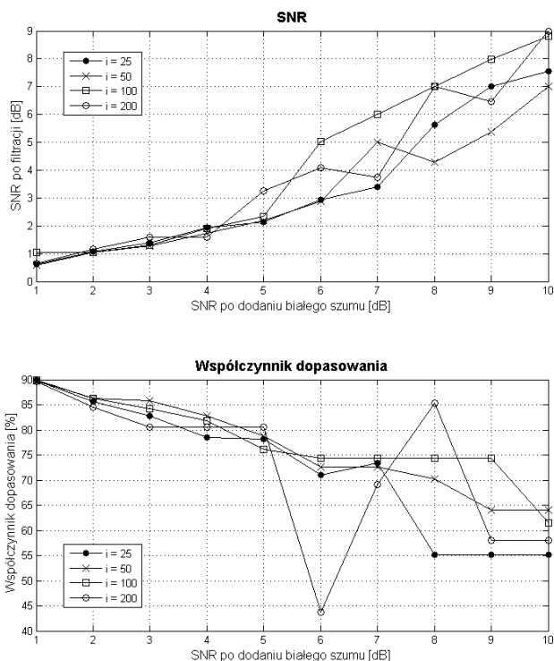
Rys 4. Przebieg SNR oraz współczynnika dopasowania fit dla różnych wartości szumu dodawanego do czystego sygnału PCG wyznaczonych dla różnych wielkości warstwy wejściowej
