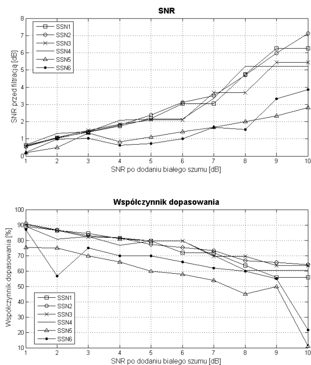
Rys 5. Przebieg SNR oraz współczynnika dopasowania fit dla różnych wartości szumu dodawanego do czystego sygnału PCG wyznaczonych dla różnych wielkości warstwy ukrytej
