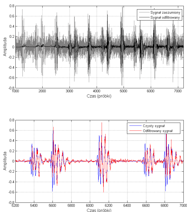
Rys 6. Wynik filtracji: A – porównanie sygnału zaszumionego z sygnałem po filtracji; oraz B – porównanie sygnału oryginalnego z sygnałem po filtracji
