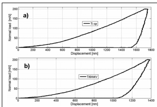
Rys. 5. Krzywe wgłębnikowania z badań na MCT: a) dla próbki z Ticip do obróbki ubytkowej, b) dla próbki Ti6Al4V z technologii DMLS
