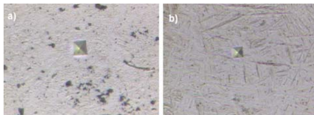
Rys. 4. Odciski wgłębnika Vickersa w próbkach: a) Ticip do obróbki ubytkowej Kavo-Everest, b) Ti64 z technologii DMLS
