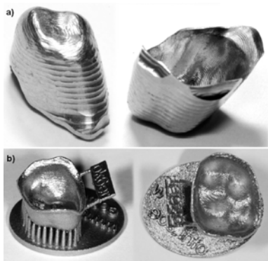
Rys.1. Podbudowy koron protetycznych wykonanych w systemie CAD/CAM: a) w technologii frezowania, b) w technologii laserowego przyrostowego spiekania
