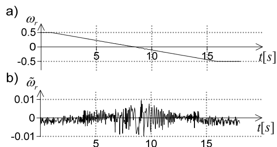
Rys.7. Wyniki badań eksperymentalnych podczas nawrotu maszyny przy zestawie wzmocnień obserwatora postaci K_0 : a) rzeczywista prędkość wirnika, b) błąd odtwarzania prędkości.
