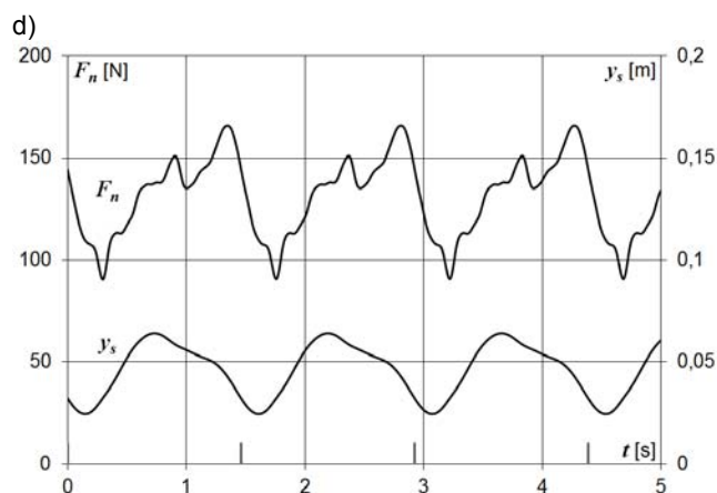
Rys.9. Wyniki symulacji układu odbierak – sieć jezdna dla modelu sieci według (5): a) dla modelu odbieraka z rys.3a; b) z rys.3b; c) z rys.4; d) z rys.5; v=160 km/h – znaczniki u dołu wykresów wskazują położenia konstrukcji wsporczych
