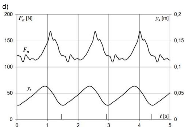
Rys.8. Wyniki symulacji układu odbierak – sieć jezdna dla modelu sieci według (4): a) dla modelu odbieraka z rys.3a; b) z rys.3b; c) z rys.4; d) z rys.5; v=160 km/h – znaczniki u dołu wykresów wskazują położenia konstrukcji wsporczych
