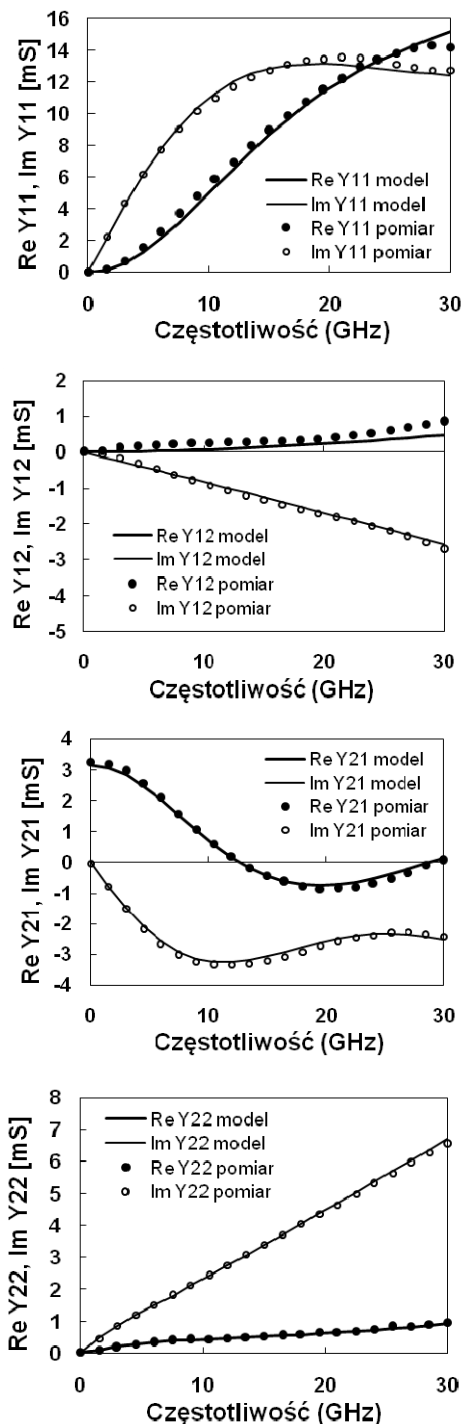
Rys. 3. Części rzeczywiste i urojone elementów macierzy admittancejnej Y_{kl} w funkcji częstotliwości. Porównanie wyników pomiarowych (pomiar) z obliczonymi (model); tranzystor MOS: W = 50 \text{ }\mu\text{m} , L = 1,4 \text{ }\mu\text{m} ; V_{DS} = 3,3 \text{ V} , V_{GS} = 1,2 \text{ V} .
