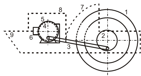
Rys. 9. Szkic rozmieszczenia urządzeń elektrowni na barce.
