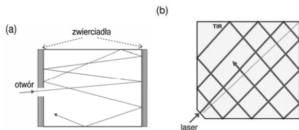
Rys. 6. Sposoby wydłużenia drogi optycznej wiązki światła wzbudzającego: a) wielokrotne odbicie przy wykorzystaniu zwierciadeł, b) wielokrotne odbicie wykorzystujące kąt graniczny {uzyskane z wykorzystaniem [7]}.
