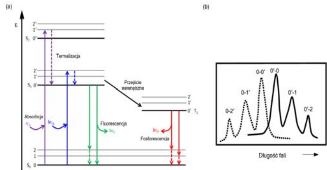
Rys. 3. Schemat poziomów elektronowych w materiałach luminescujących (a) oraz widmo luminescencji będące wynikiem przejść singletowych i oscylacyjnych (b). Z lewej strony pokazany jest schemat Jabłońskiego, z prawej widmo absorpcyjne (linia przerywana) i widmo emisyjne (linia ciągła) wynikające z schematu Jabłońskiego, z włączeniem struktury oscylacyjnej.
