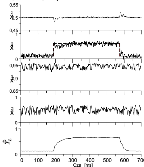
Rys.5. Zmiana momentu obciążenia do około 0,6 j.w.
