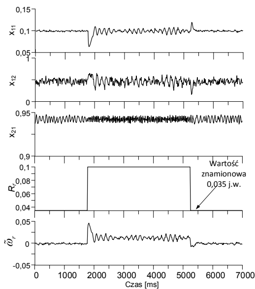
Rys.8. Zmiana rezystancji wirnika z 0,035 na 0,1 j.w., maszyna obciążona momentem o wartości 0,45 j.w.
