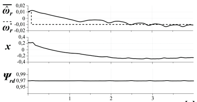
Rys.10. Nawrót silnika od 0,01 do -0,01 j.w. przy uszkodzeniu fazy A
