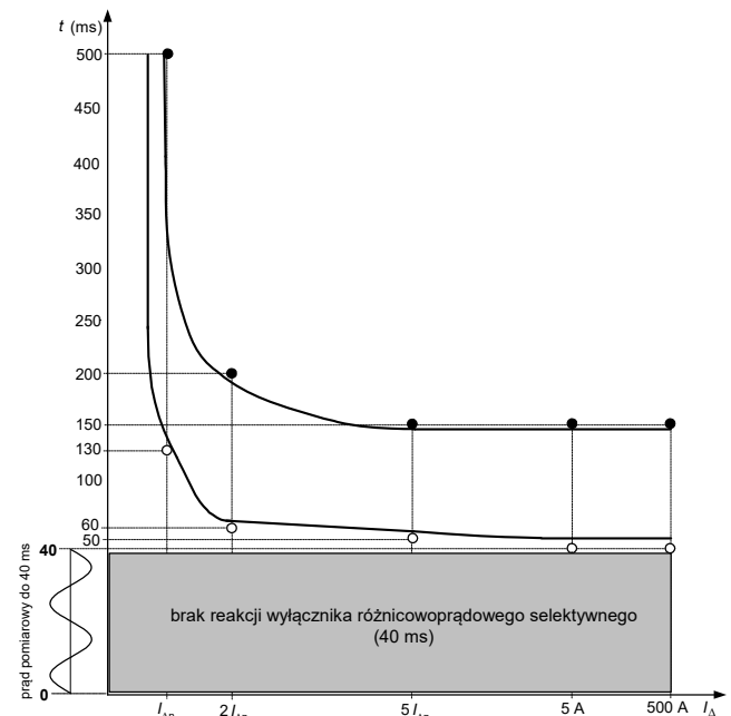
Rys.4. Charakterystyka czasowo-prądowa wyłącznika różnicowoprądowego selektywnego
