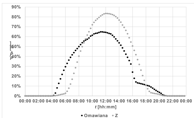
Rys.4. Nałożenie na siebie krzywych generacji mocy omawianej instalacji oraz instalacji z lokalizacji Z (jako krzywej „idealnej”)
