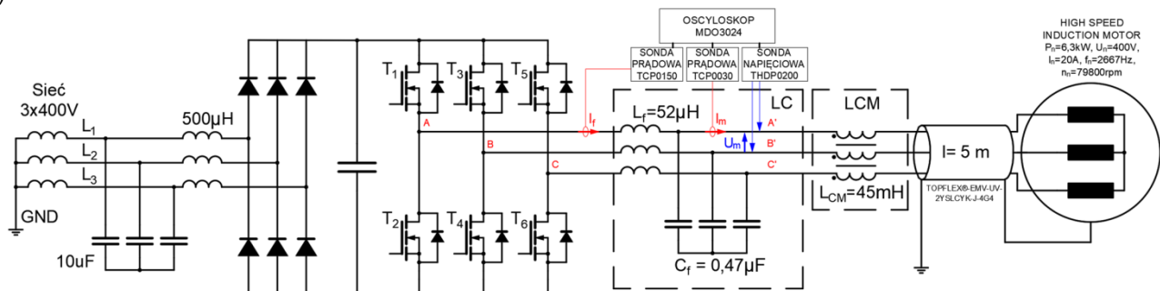
Rys. 6. Opracowane stanowisko badawcze z wysokoobrotowym silnikiem indukcyjnym zasilanym z falownika SiC oraz umieszczonym na wspólnym wale wysokoobrotowym silnikiem PMSM modelującym obciążenie turbosprężarką powietrza ogniwa paliwowego
