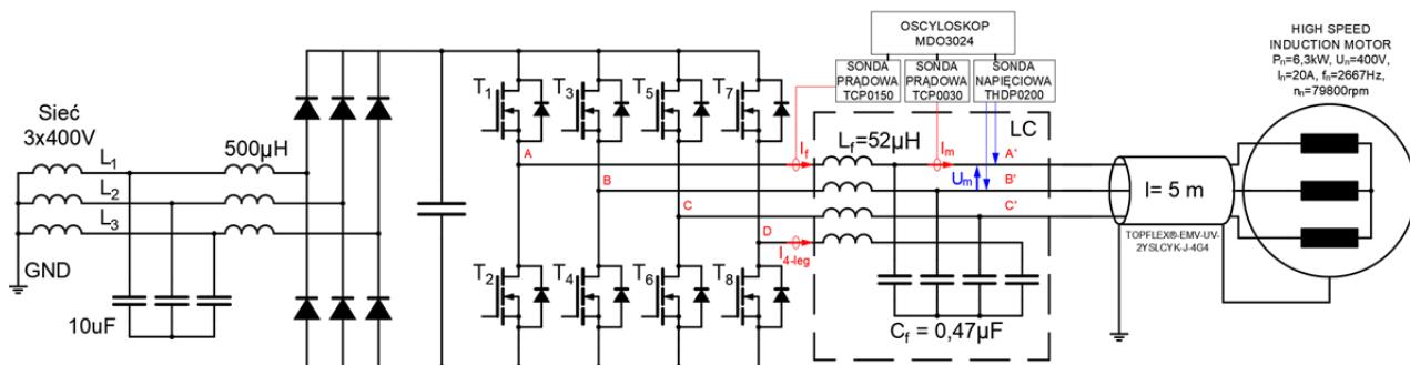
Rys. 7. Schematy badanego stanowiska w dwóch konfiguracjach: z falownikiem 3-galeziowym i dławikiem L_{CM} = 45 mH (a) oraz w konfiguracji z falownikiem 4-galeziowym bez dławika L_{CM}
