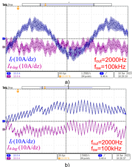
Rys. 11. Przebiegi prądu I_f 4-gałęzi fazy oraz prądu czwartej gałęzi I_{4-leg} przy sterowaniu z modulacją CMRM (bez dławika L_{CM} ) przy prędkości obrotowej silnika 60 000 obr/min (a); zarejestrowana występująca w niektórych sektorach zwiększona częstotliwość przełączeń czwartej gałęzi (b)
