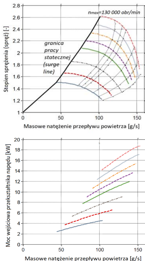
Rys.1. Mapy wydajności turbosprężarki ogniwa paliwowego 100 kW
