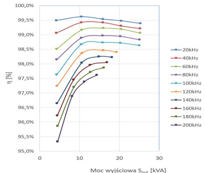
Rys. 4. Sprawność opracowanego falownika SiC w funkcji częstotliwości przełączania tranzystorów f_{sw}
