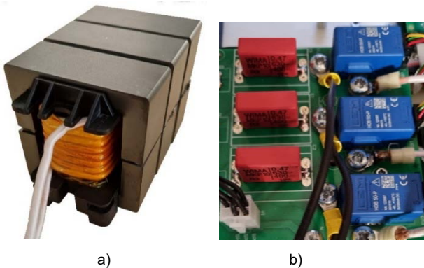
Rys. 5. Widok zaprojektowanego dławika z rdzeniem ferrytowym (a) oraz kondensatorów filtra sinusoidalnego LC
