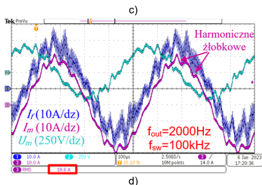
Rys. 10. Przebiegi prądu I_f falownika SiC, prądu silnika I_m oraz napięcia międzyprzewodowego U_m za filtrem sinusoidalnym przy prędkości 60 000 obr/min ( f_{out} = 2 kHz): falownik SiC 3-gałęziowy z modulacją SVPWM i dławikiem L_{CM} = 45 mH przy biegu jałowym (a) i obciążonym silniku (b); falownik 4-gałęziowy z modulacją CMRM (bez dławika L_{CM} ) przy biegu jałowym (c) i przy obciążeniu (d)
