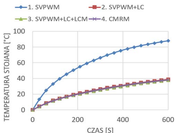
Rys. 8. Przyrost temperatury stojana badanego wysokoobrotowego silnika indukcyjnego HS-IM w zależności od metody modulacji falownika i zastosowania bądź nie filtra LC oraz filtra CM
